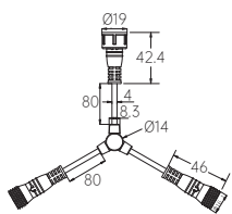
Y型4位连接件
