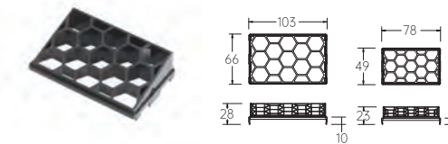
迷你景观洗墙灯系列蜂窝配件
