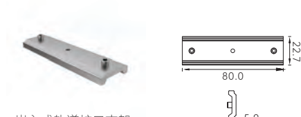
嵌入式轨道扩口支架
