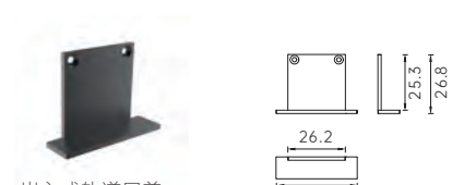
嵌入式轨道尾盖
