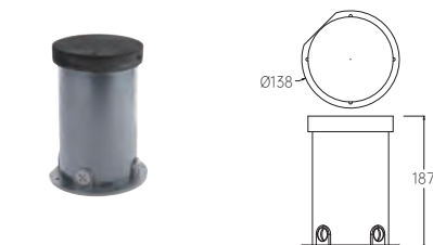
景观灯地面安装盖
