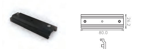
标准明装轨道扩口支架
