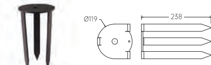
不锈钢景观灯安装地插
