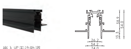
嵌入式无边轨道
